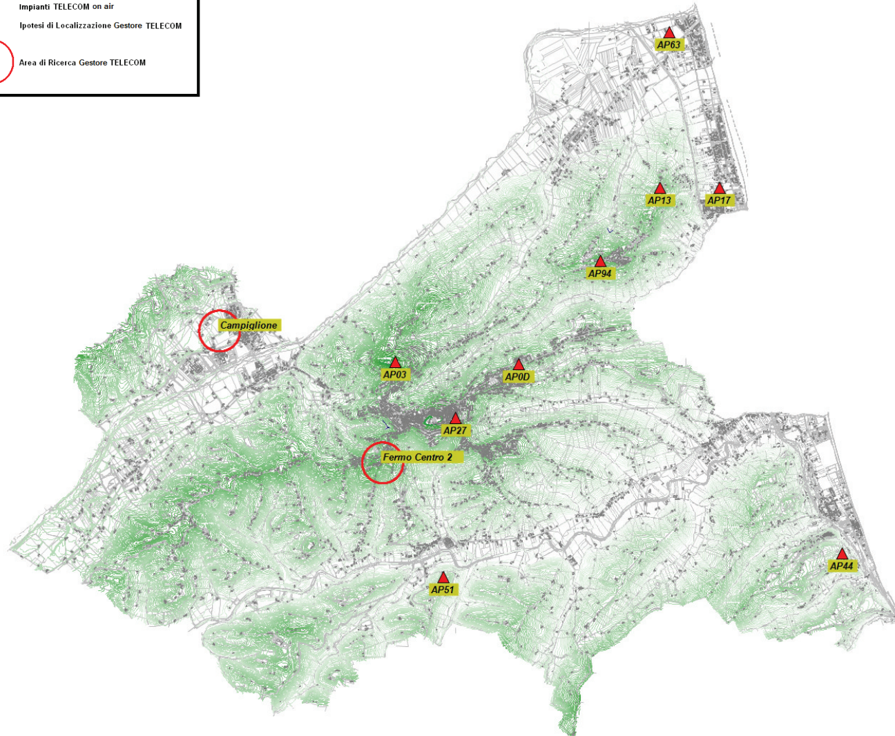
Fig. 22 Piano di rete - Gestore TELECOM
